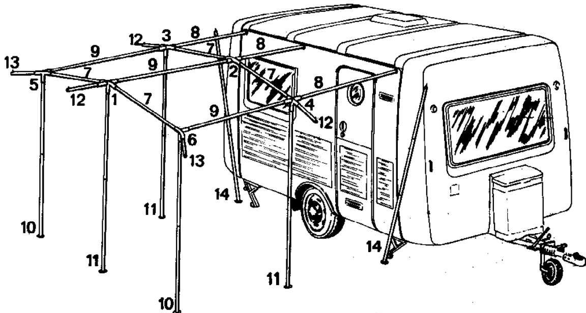
Abb. 25 Vorzeltgestänge
